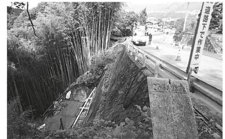
工事が進む佐原線 最終工区の土留工に着手（この工事は一部を債務負担として発注されている）
