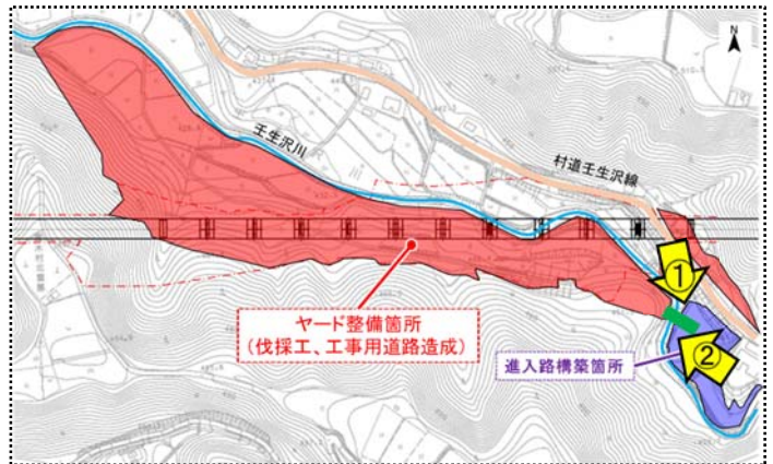
壬生沢高架橋区間 (ヤード整備箇所)
