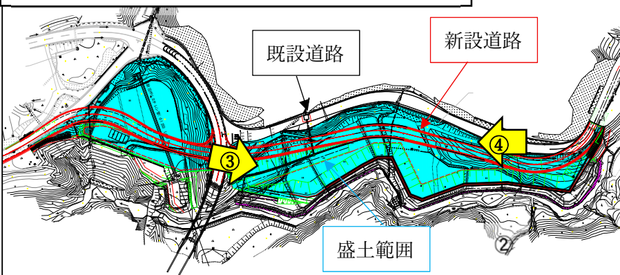
壬生沢線道路改良工事 (開田・鬼の久保)
