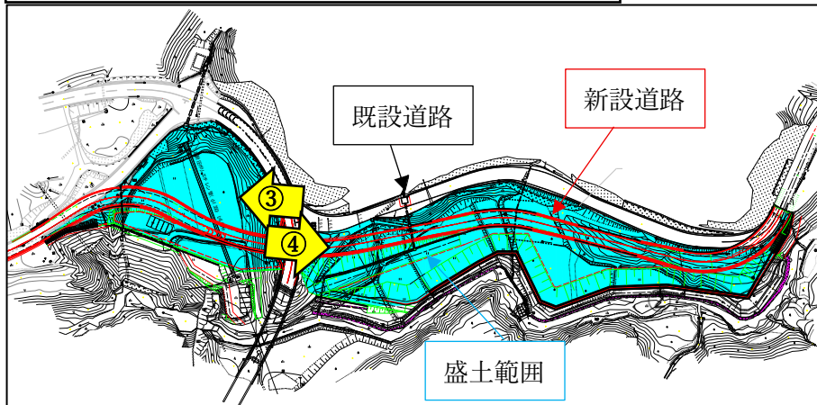
壬生沢線道路改良工事 (開田・鬼の久保)
