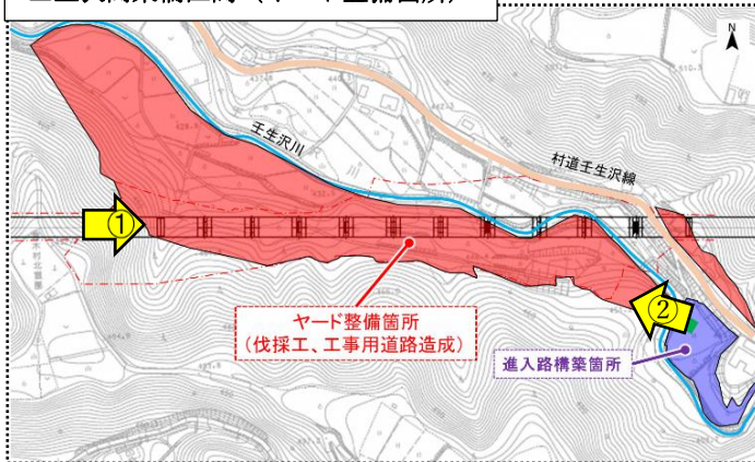
壬生沢高架橋区間 (ヤード整備箇所)
